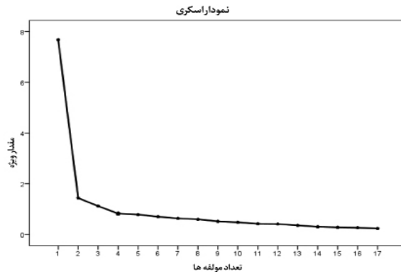
جدول ۱: نمودار سنگ‌ریزه به منظور تشخیص تعداد عامل‌ها
